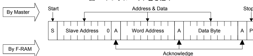
図 7. シングルバイト書き込み
