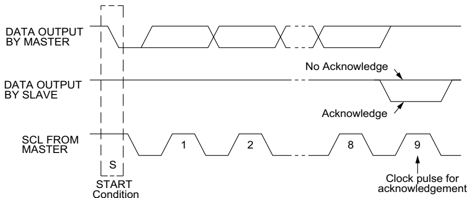
図 5. I 2 C バス上のアクノリッジ
